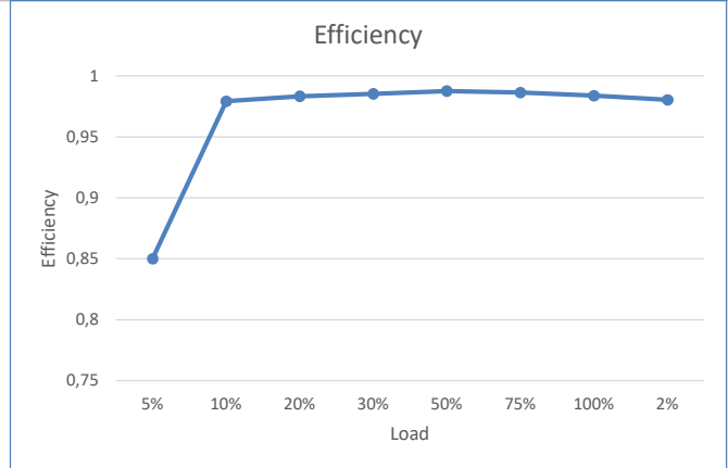
Verimlilik Eğrisi
